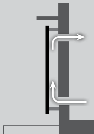
Muro Trombe-Michel
